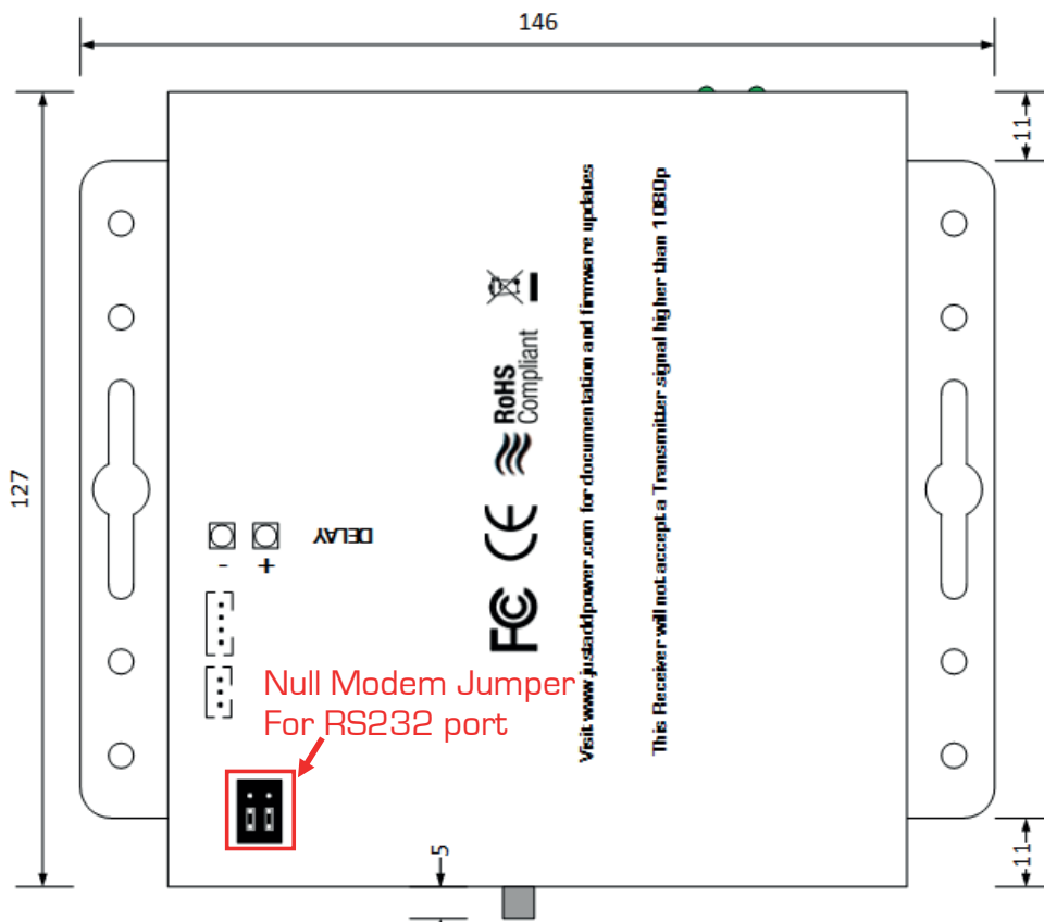
515PoE Bottom
