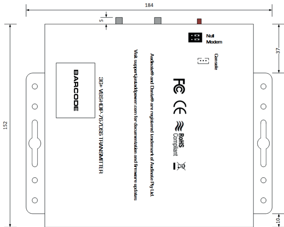
767DSS Bottom
